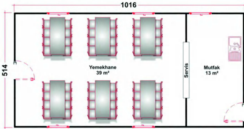
• 52 m² Prefabrik Yemekhane
