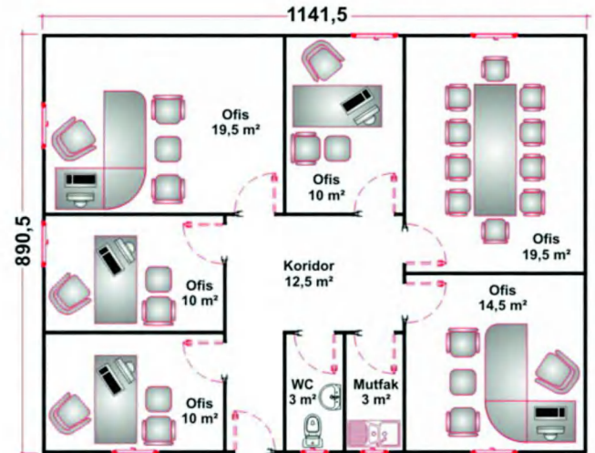
• 102 m 2 Prefabrik Ofis
