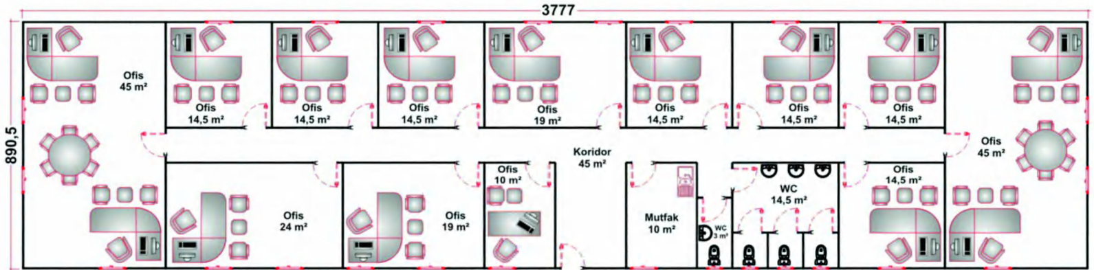
• 336 m 2 Prefabrik Ofis
