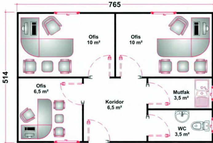
• 39 m 2 Prefabrik Ofis
