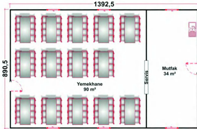
• 124 m² Prefabrik Yemekhane
