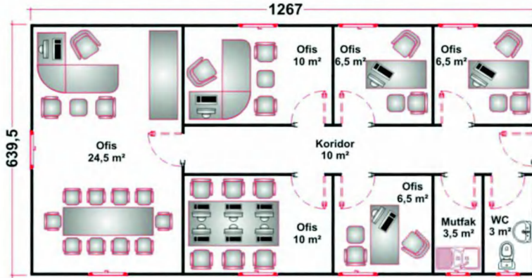
• 81 m² Prefabrik Ofis
