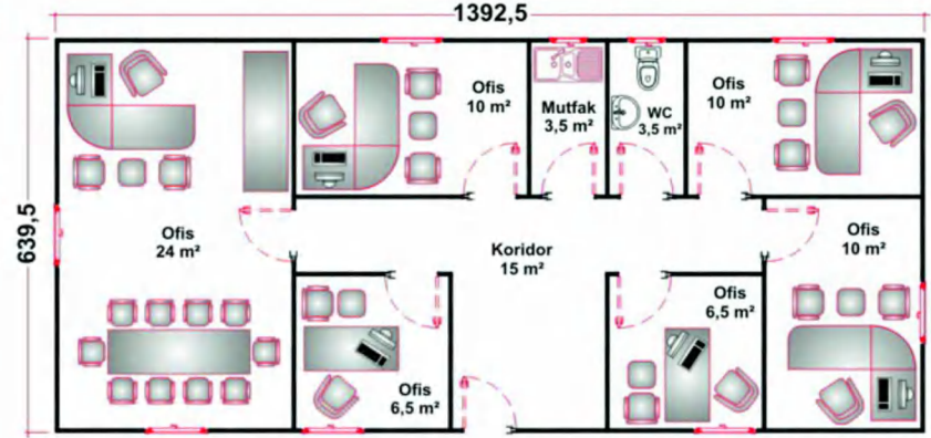
• 89 m² Prefabrik Ofis
