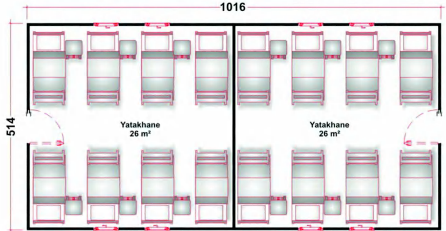
• 52 m² Prefabrik Yatakhane
