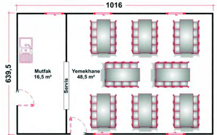
• 65 m² Prefabrik Yemekhane
