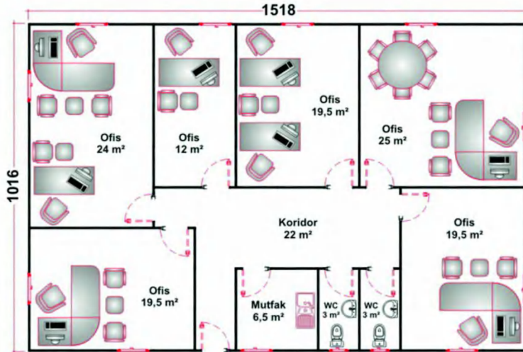
• 154 m² Prefabrik Ofis
